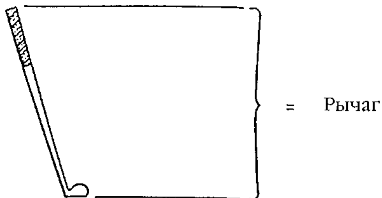
Рисунок 8-6 Пример рычага
