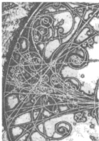
Треки элементарных частиц в пузырьковой камере
