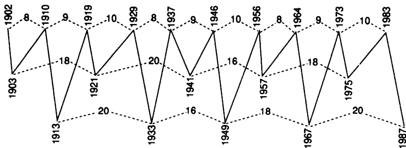
Циклический график Беннера–Фибоначчи
