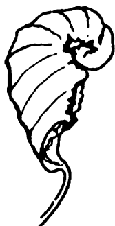
Засыхающий лист пойнсеттии
